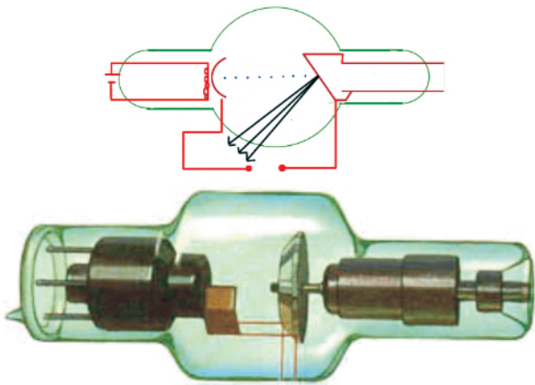
图10 基于韧致辐射原理的 X 射线管之原理图与实物图 来自阴极(左侧)的热发射电子被加速, 入射到金属阳极内部被骤然减速, 发出连续谱的 X 射线
