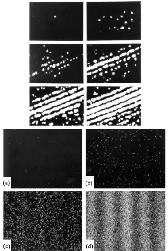
图6 (上图)1974年完成的由直接电视屏所得到的一组电流不断加大的干涉图像.6幅小图的积分时间都是0.04s.由于每一时刻只有一个电子打到屏幕上,这些图显示了如何由单电子行为获得干涉图像(下图)1989年Akira Tonomura及其合作者获得的双缝干涉图像(a)8;(b)270;(c)2000;(d)60000个电子 [10]
