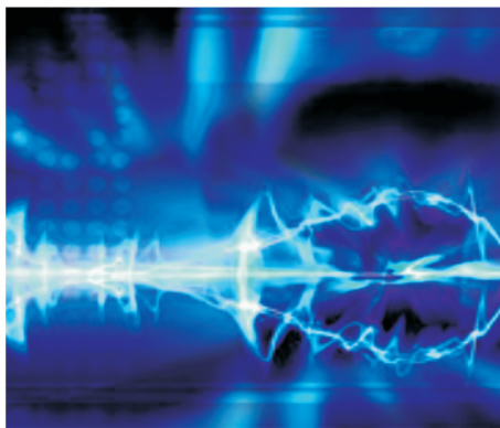
图4 电子 Zitterbewegung 的假想图. 该运动一直未能被确立为物理学的实在
