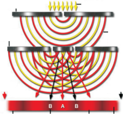
图5 杨氏双缝干涉实验.其实验结果为一组明暗相间的条纹.关于条纹的细节,一般文献都语焉不详
